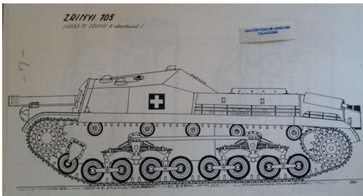
10. képmelléklet: A 105 milliméteres 40M tarackkal szerelt Zrínyi-II rohamlöveg tervrajza 638
